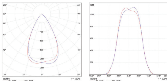
60° 3000K
